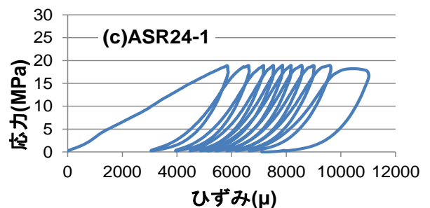
図 3-4 応力—ひずみ関係
