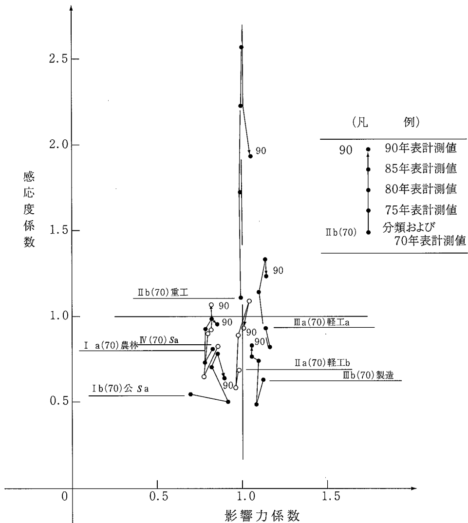
【図7】影響力係数と感応度係数の経年変化 1970-90年
